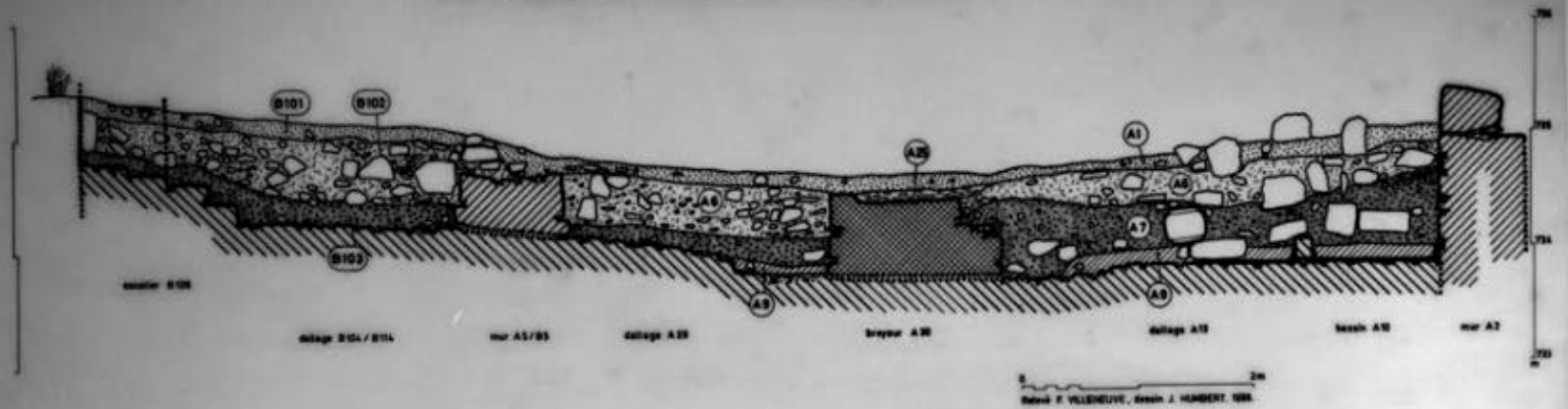
KHIRBET_EDH_DHARIH, Village. Huilerie V10. Coupe stratigraphique est-ouest dans l'axe du bâtiment.
